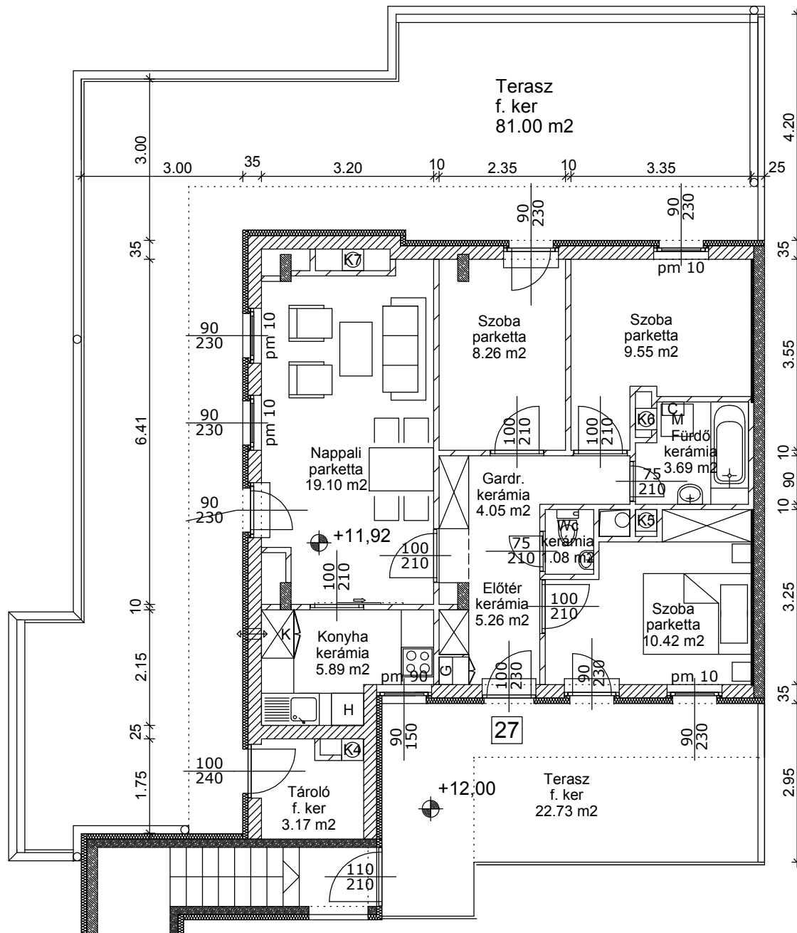
TETŐTÉR 27. LAKÁS M 1:100
