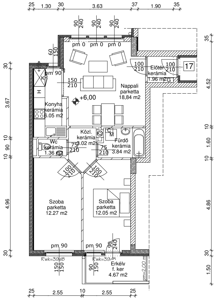
EMELET 17. LAKÁS M 1:100
