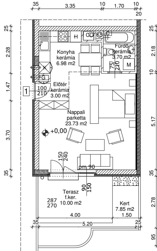
FÖLDSZINT 01. LAKÁS M 1:100
